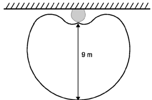
Erfassungsbereich des Glasbruchsensors
